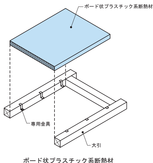
ボード状プラスチック系断熱材
