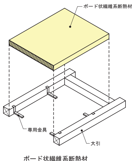
ボード状繊維系断熱材
